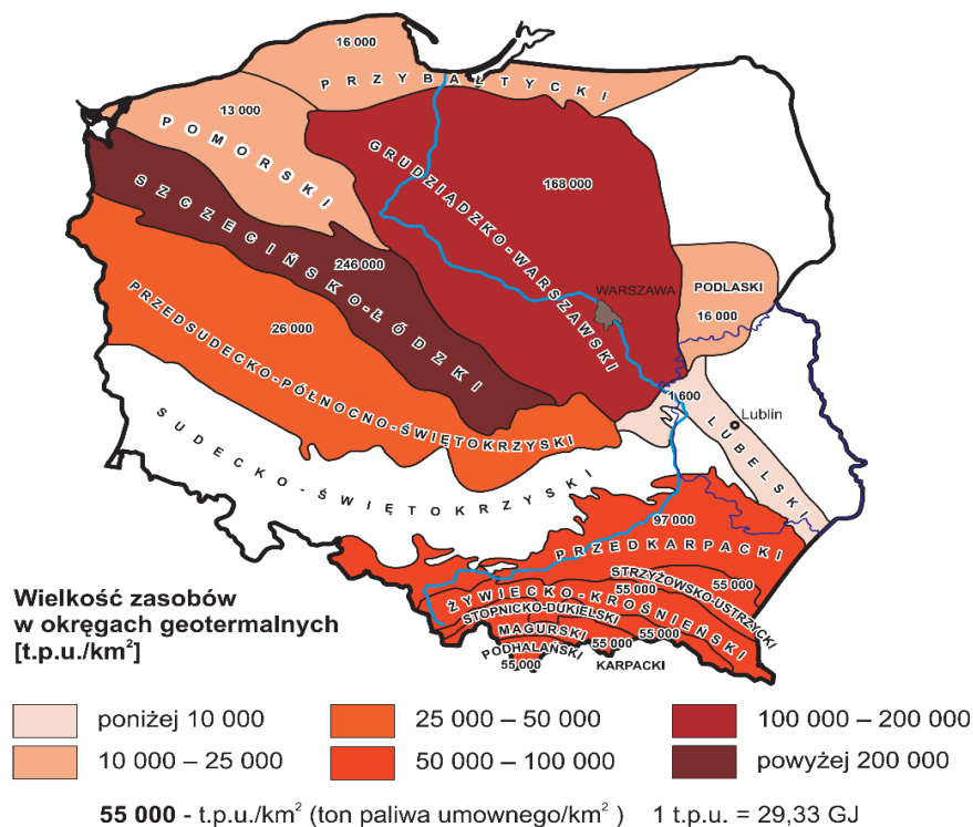
Mapa 8. Zasoby energii geotermalnej w Polsce.
