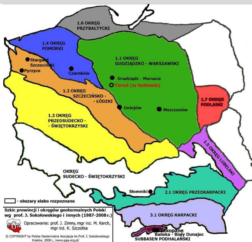
Mapa 7. Szkic okęgów geotermalnych Polski.
