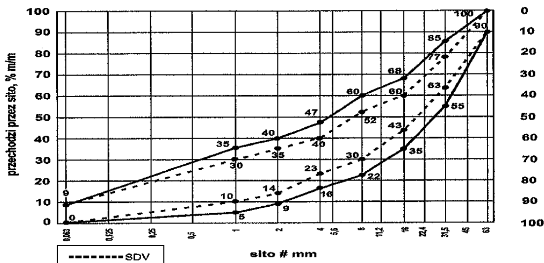
Rys. 3. Krzywe graniczne uziarnienia mieszanki kruszywa niezwiązanego 31,5/63 mm do warstw podbudowy zasadniczej
